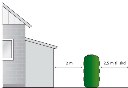
Plasttanke placeret i det fri:
